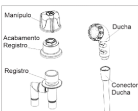
Instalação sem aquecedor
