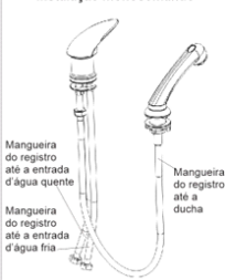
Instalação monocomando
